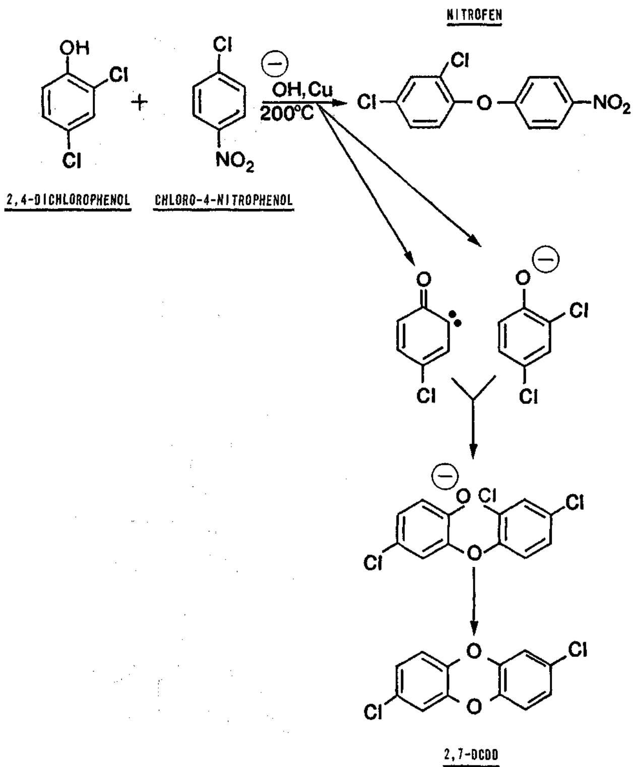
Figure 21. Nitrofen.
