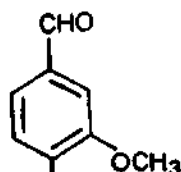
(25) VANILLIN
